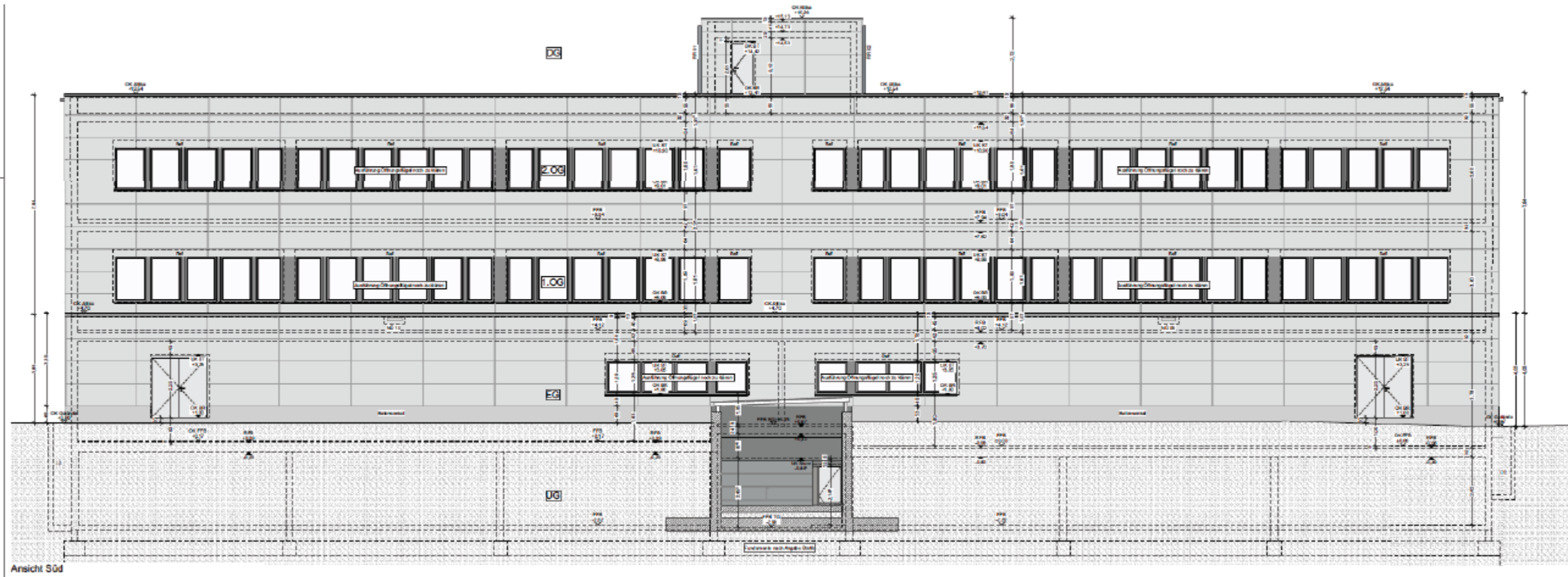
Ansicht Süd
